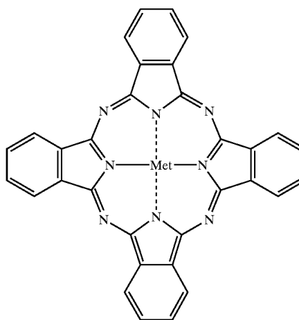
Met-Pc
