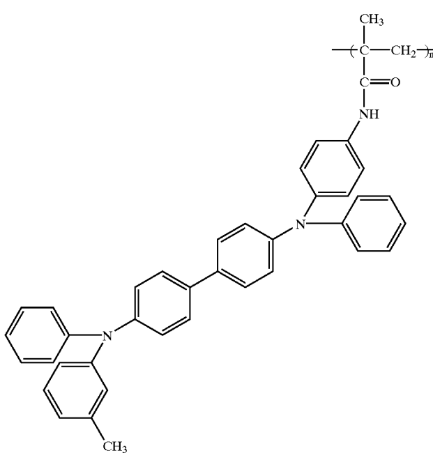
TPD-PMAA
