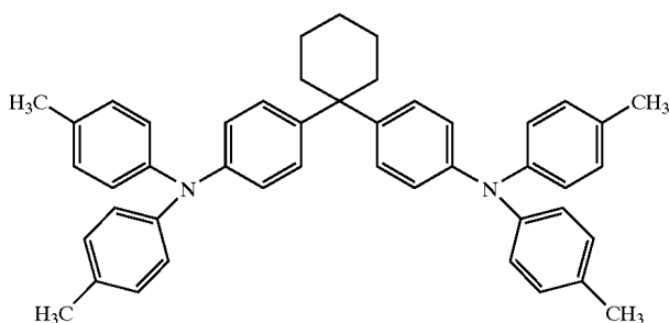
TPAC
