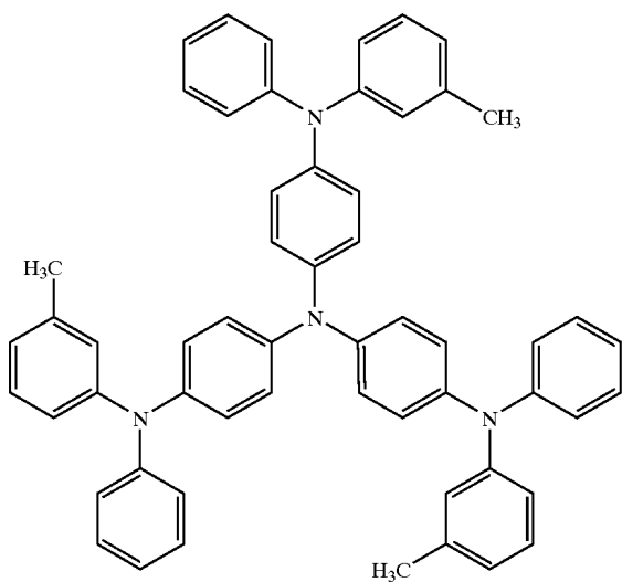
m-MTDATA
