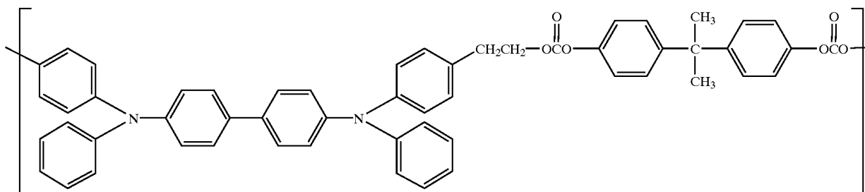
TPD-PCA
